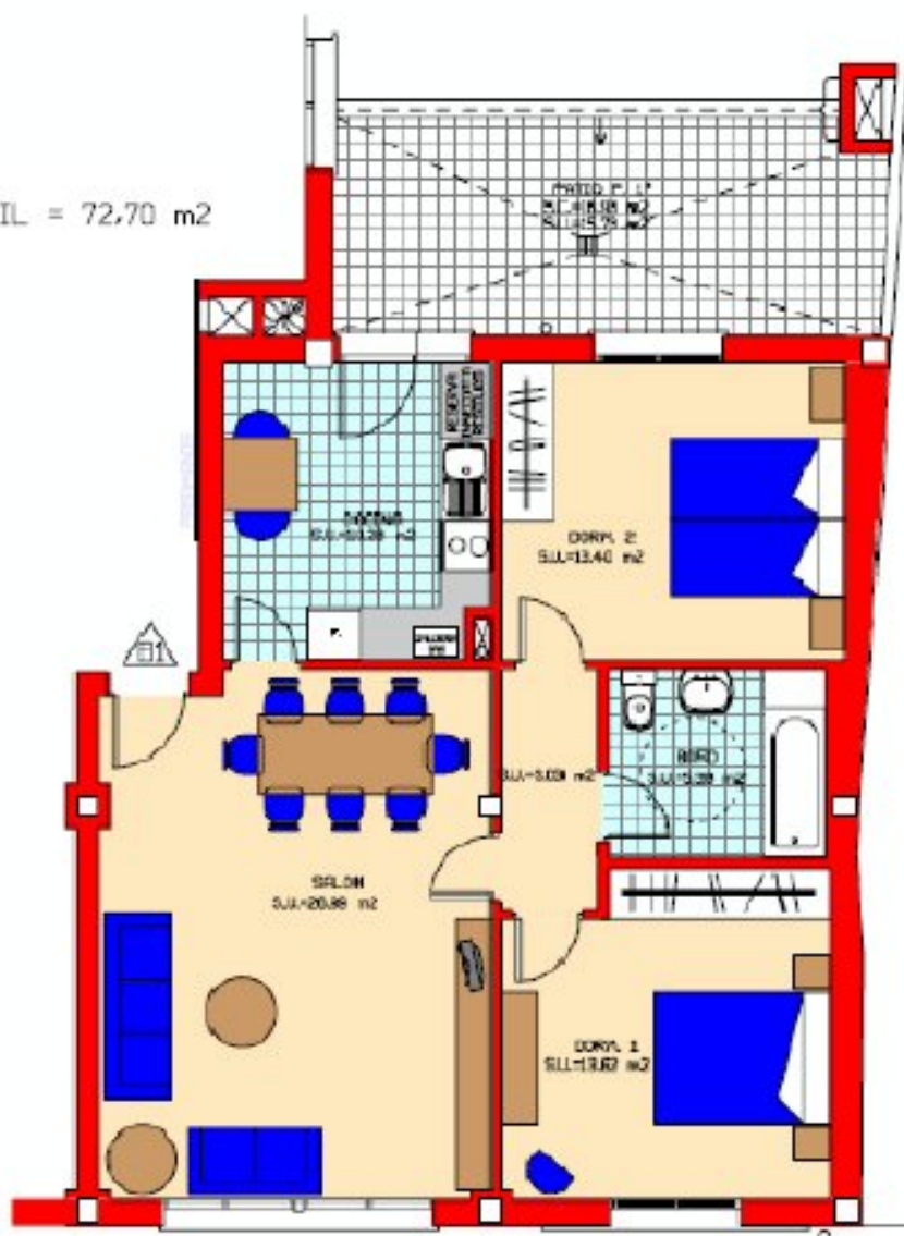
PLANTA PRIMERA
